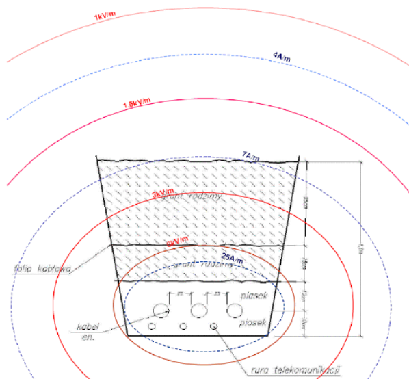
Rys. Rozkład pola elektromagnetycznego nad projektowaną linią kablową (kolorem czerwonym oznaczono izolację pola elektrycznego, kolorem niebieskim – izolację pola magnetycznego)
